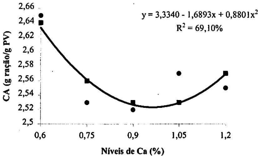
FIGURA 3. Efeito dos níveis de cálcio dentro da granulometria grossa do calcário (DGM=0,899mm) sobre a conversão alimentar no período de 3 a 5 semanas de idade.
